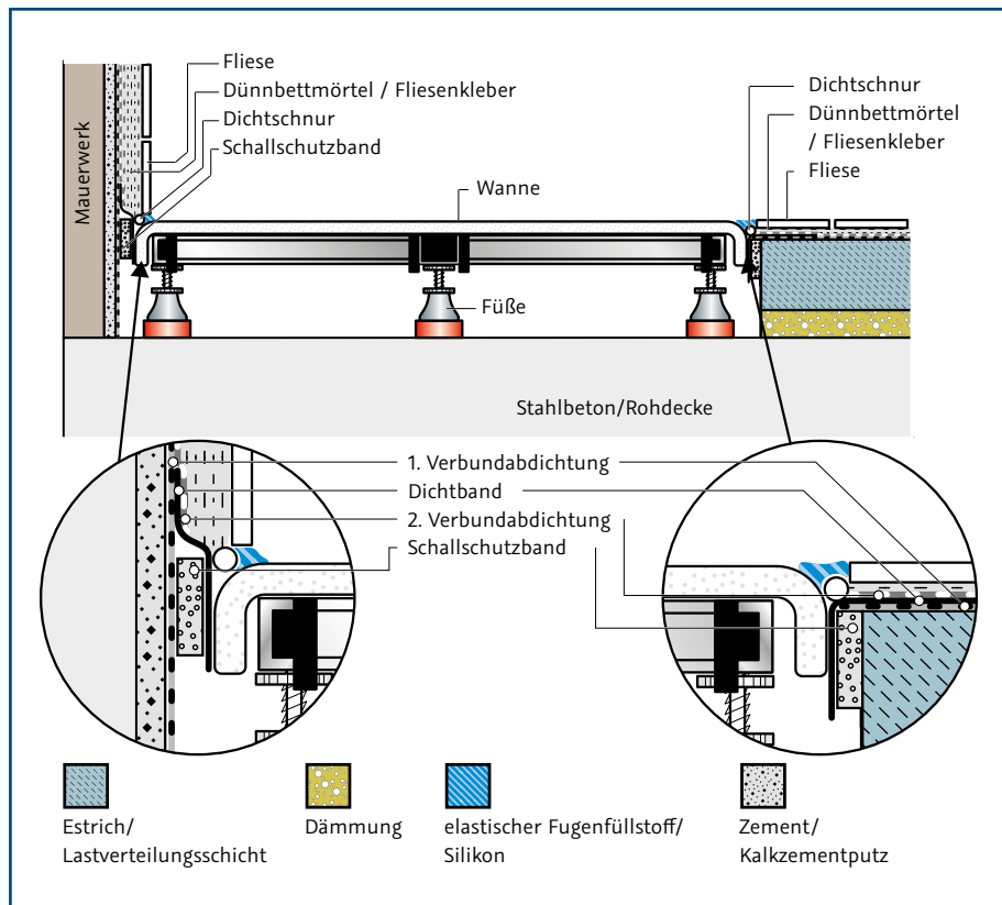
Automatischer Ausgleich der Wannenebenen durch federgelagerte und klebefixierte Stifte.
