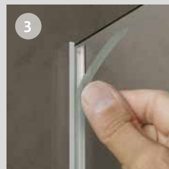
Scheibe fixieren und abdichten
