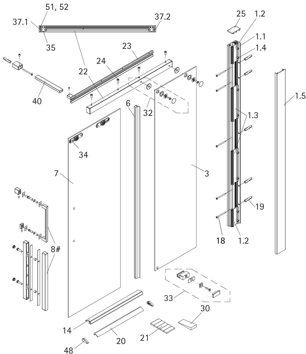
Abb.: Festelement links, Türseite rechts
