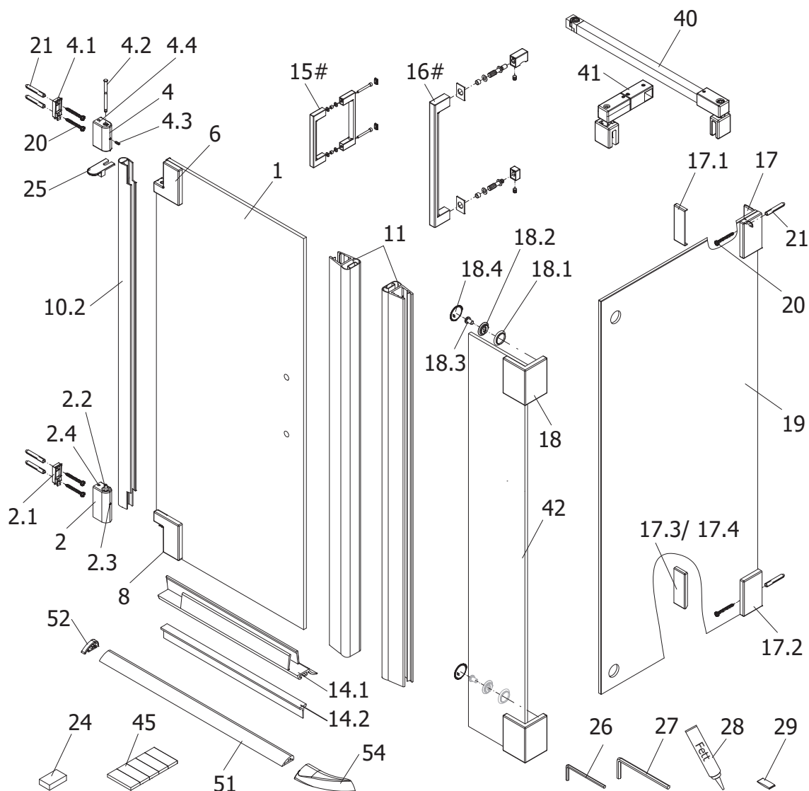
Abb.: Anschlag links
